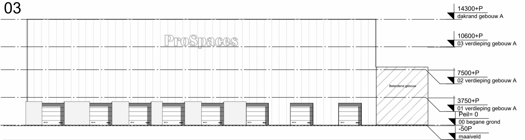
Achtergevel verkoop
