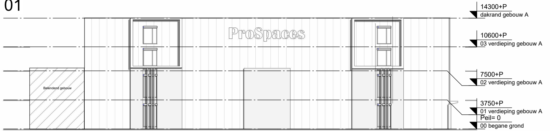
Voorgevel verkoop
