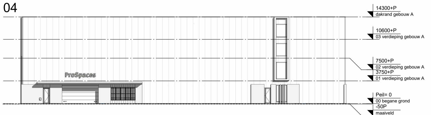
Rechtergevel verkoop
