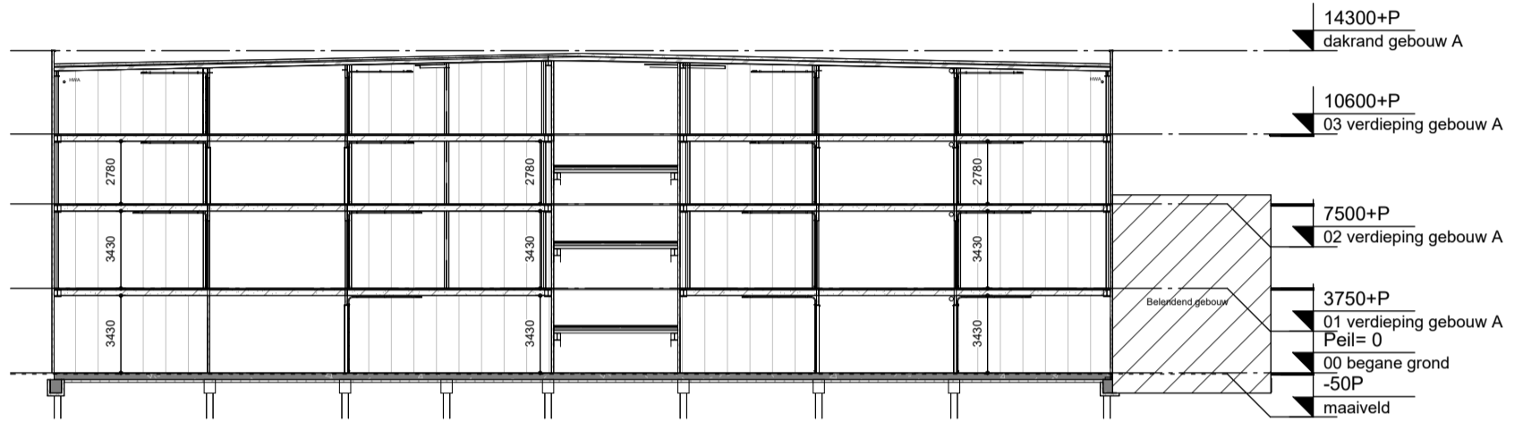
Doorsnede B-B
