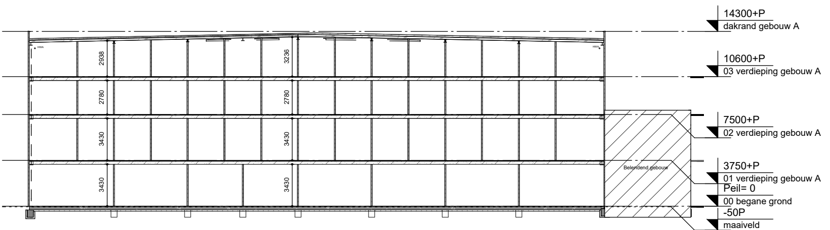
Doorsnede C-C
