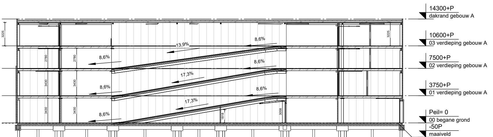
Doorsnede D-D
