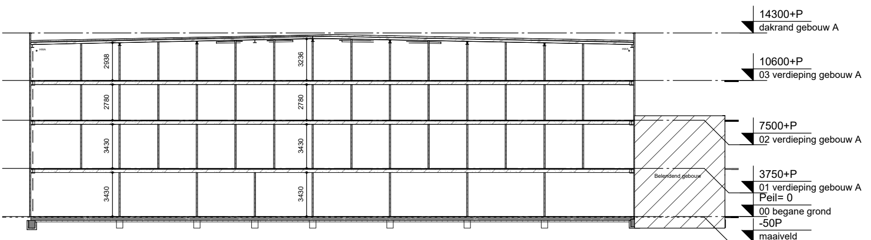
Doorsnede C-C
