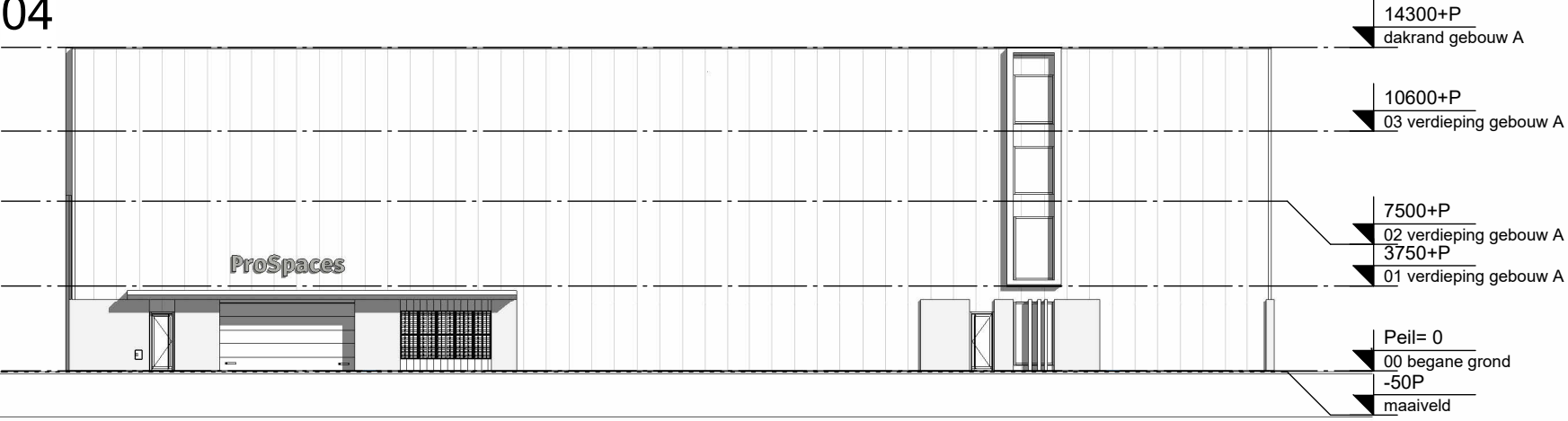
Rechtergevel verkoop
