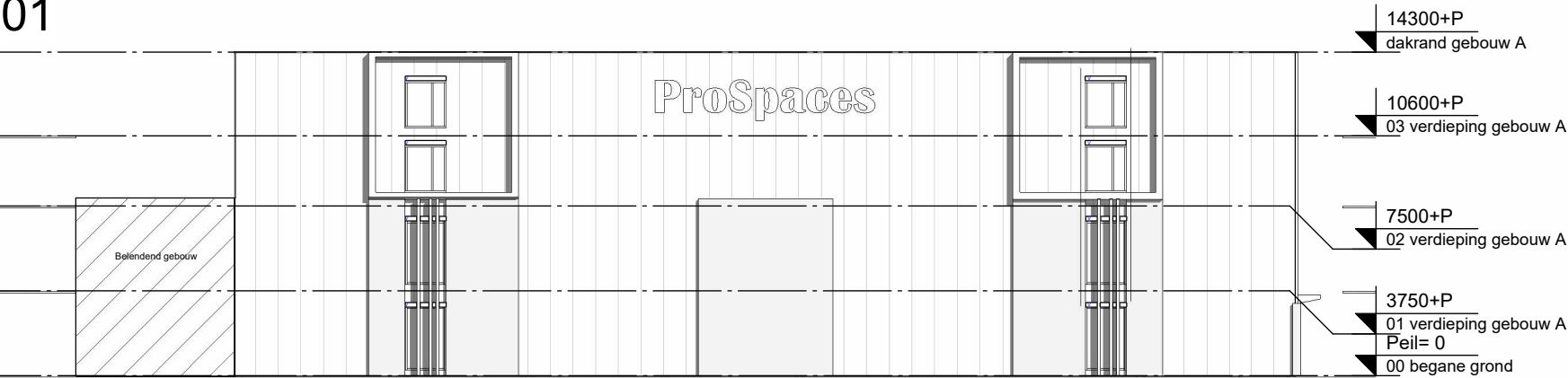
Voorgevel verkoop
