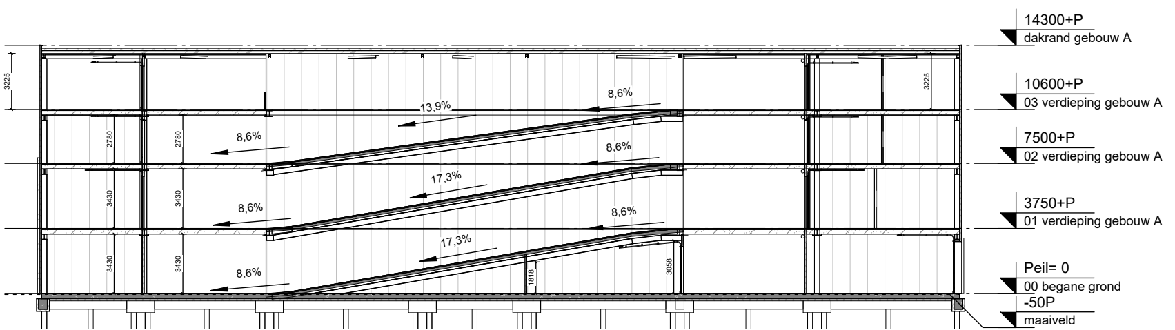
Doorsnede C-C
