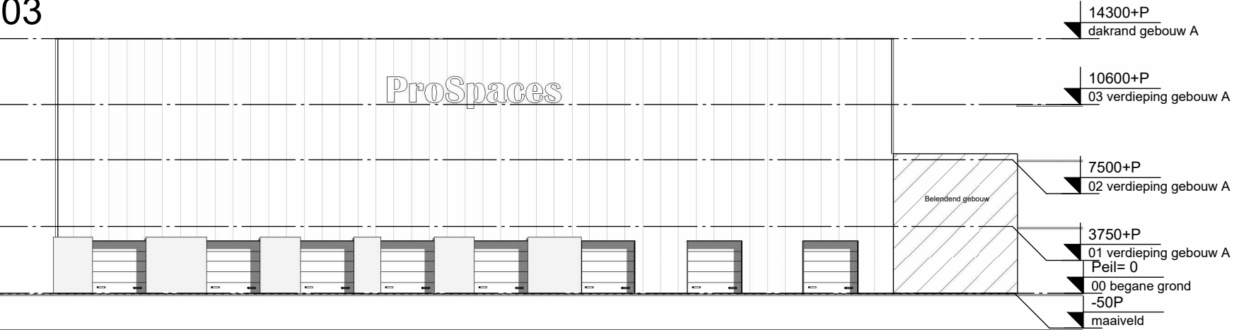
Achtergevel verkoop
