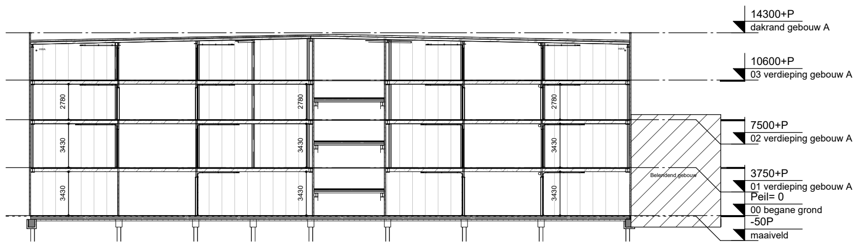
Doorsnede B-B
