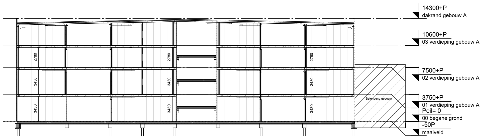
Doorsnede B-B
