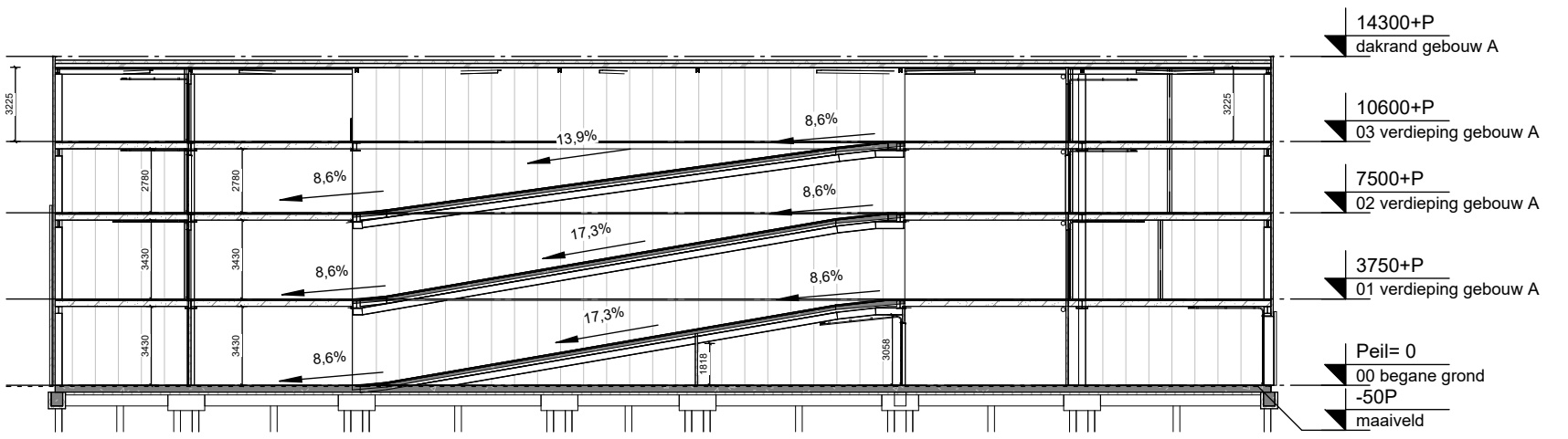
Doorsnede C-C
