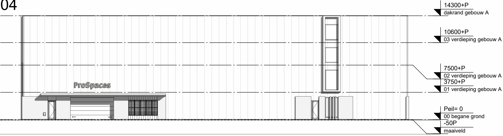
Rechtergevel verkoop
