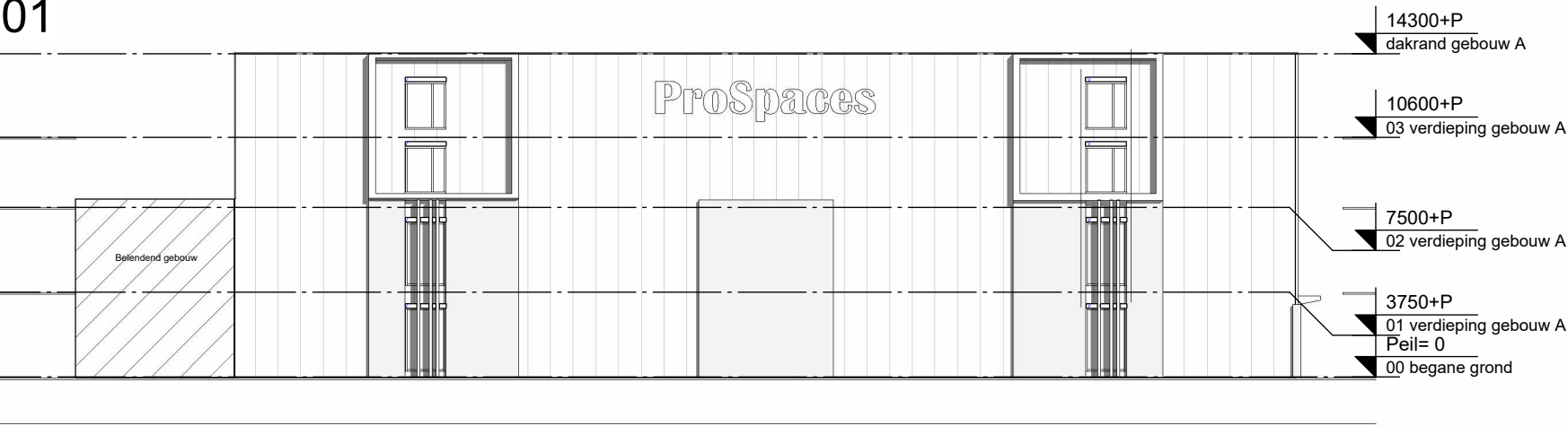
Voorgevel verkoop
