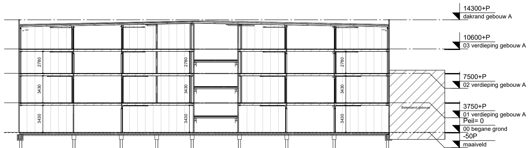
Doorsnede B-B
