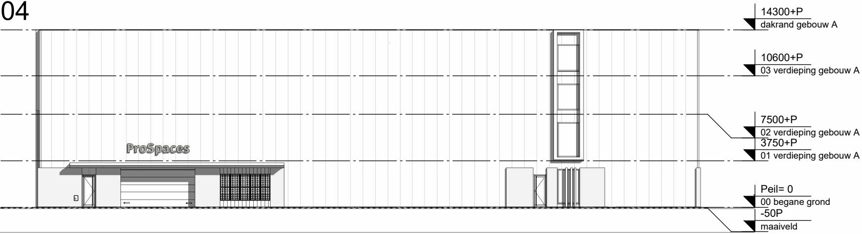
Rechtergevel verkoop
