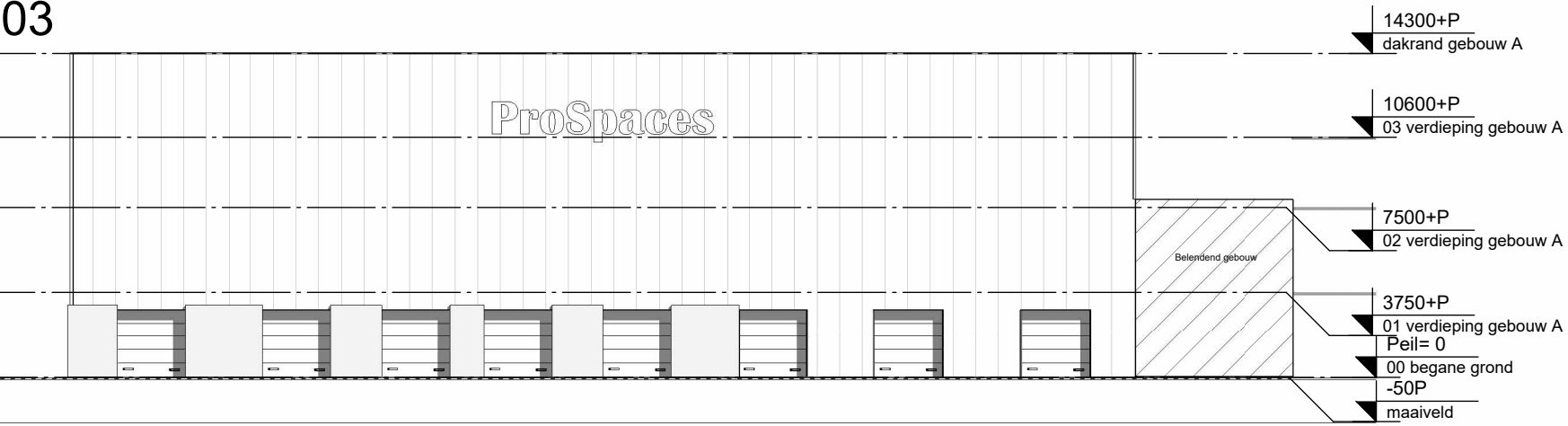
Achtergevel verkoop
