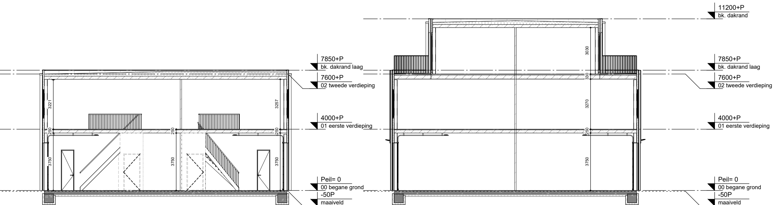
Doorsnede A-A
