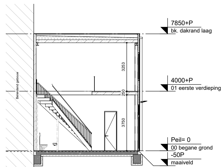
Doorsnede B-B
