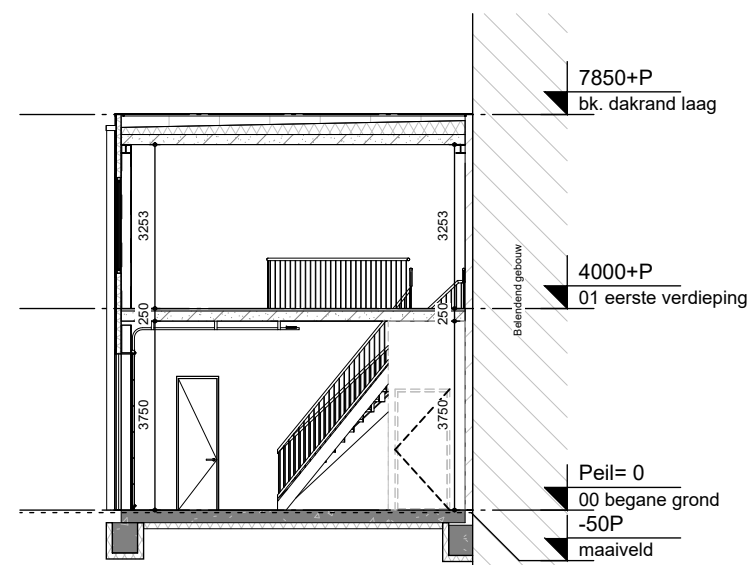
Doorsnede A-A
