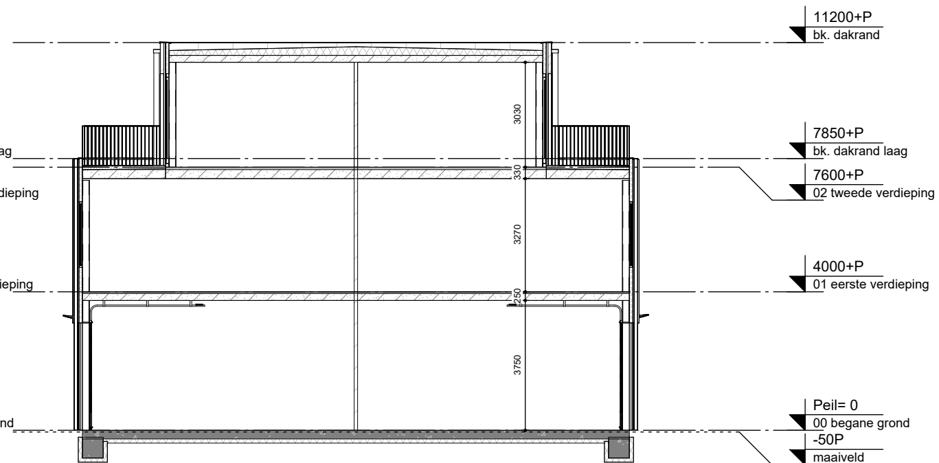
Doorsnede B-B
