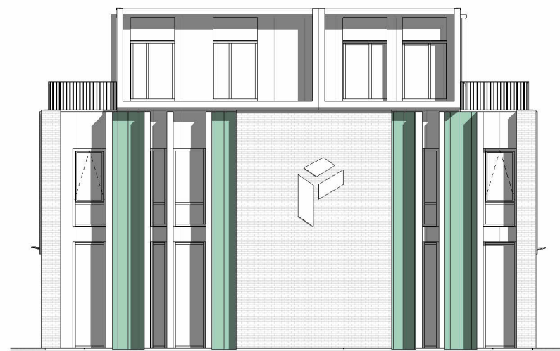
Rechtergevel gebouw B
