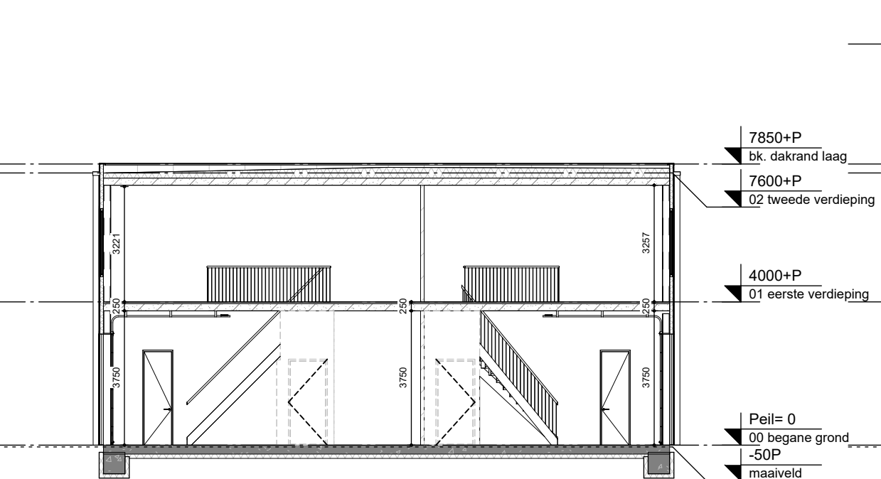
Doorsnede A-A
